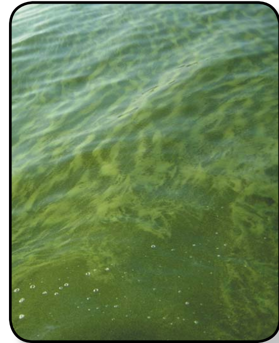
Fleur d'eau de cyanobactéries. Les cyanobactéries sont en suspension dans les eaux du lac.
